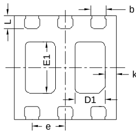
Bottom View 背面视图
